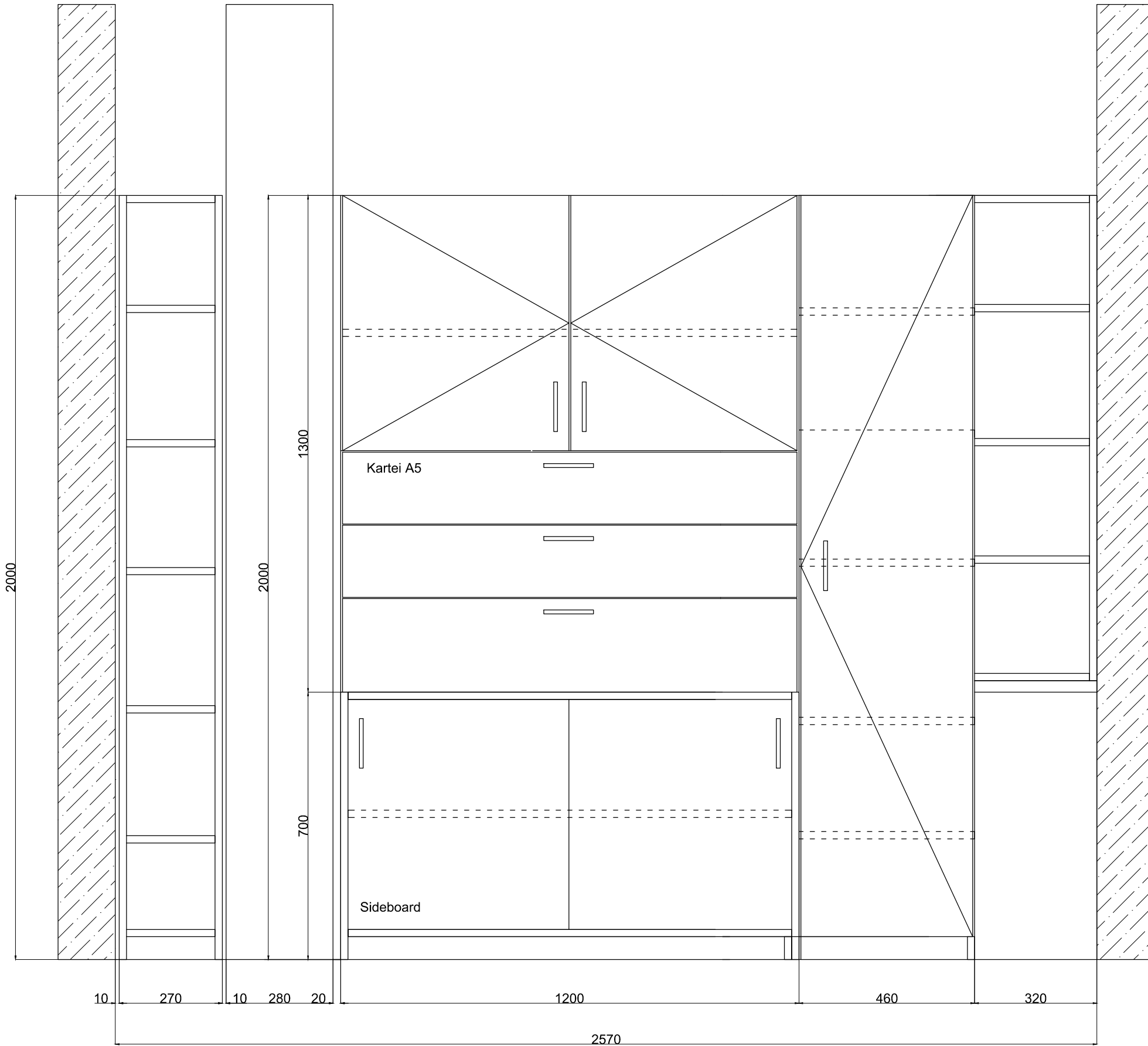
Ansicht Schränke
